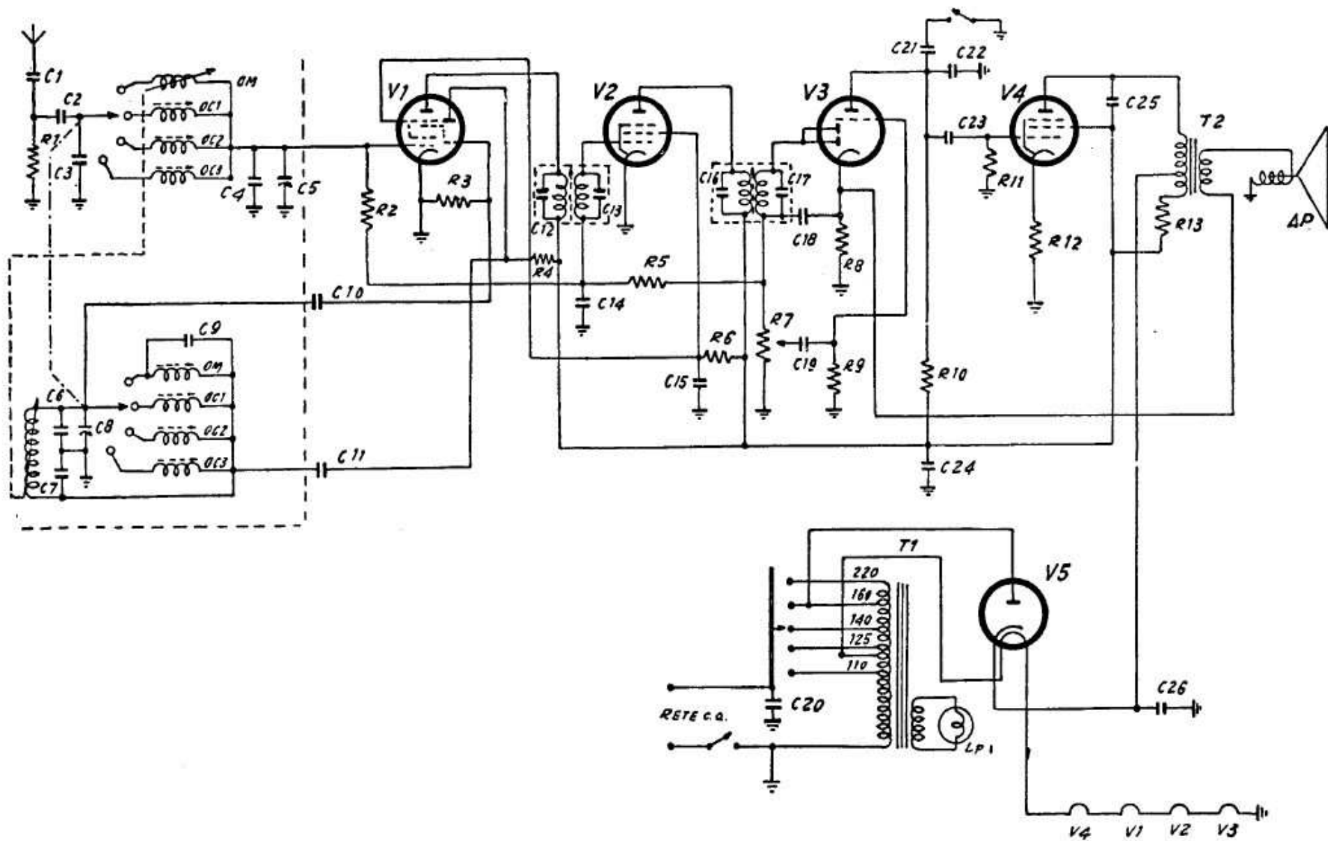
ALLOCCIO BACCHINI - Mod. 425. Apparecchio di piccole dimensioni, ad onde medie e tre bande onde corte. Media frequenza 465 kc/s. (Vedi a pag. 18 le tabelle dei valori e di taratura).
